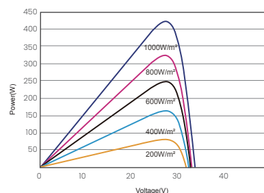
昊宇光伏P-V曲线图(425W)
