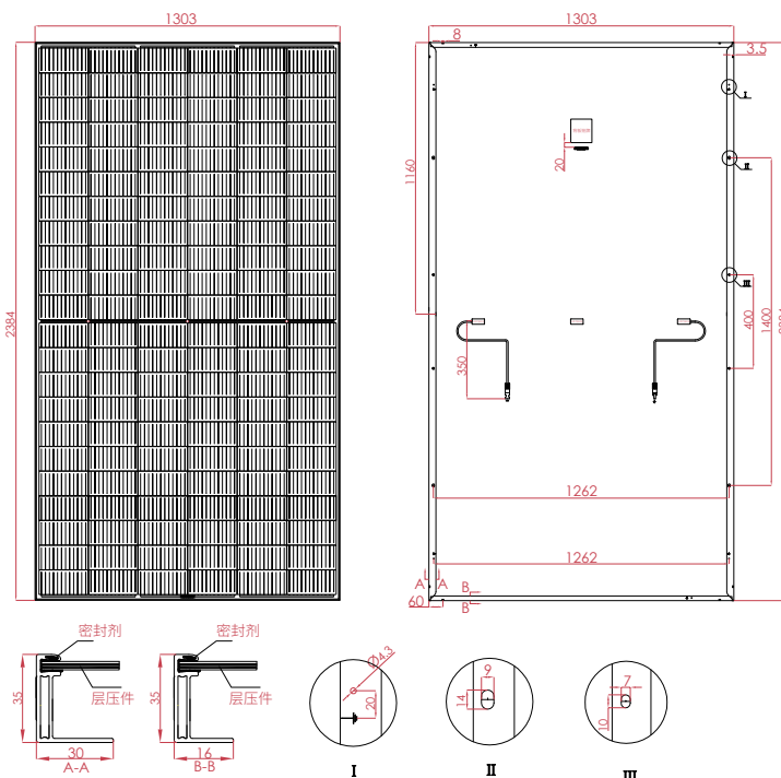
工程图纸
