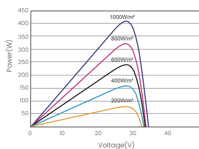
昊宇光伏P-V曲线图(405W)
