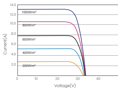
昊宇光伏I-V曲线图(405W)
