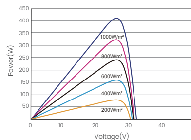
昊宇光伏P-V曲线图(410W)
