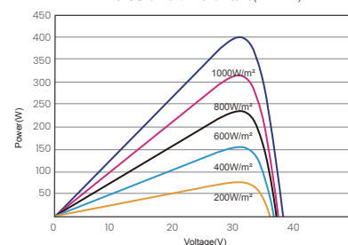
昊宇光伏P-V曲线图(400W)
