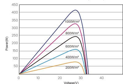
昊宇光伏P-V曲线图(410W)
