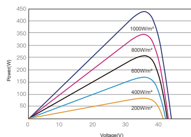
昊宇光伏P-V曲线图 (445W)
