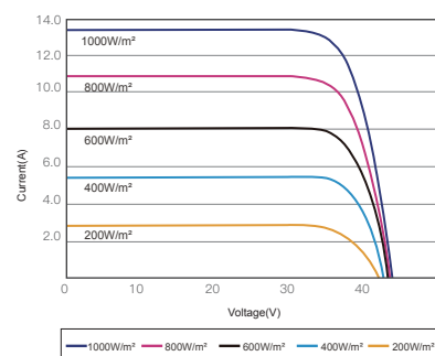
昊宇光伏I-V曲线图 (445W)
