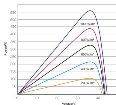
昊宇光伏P-V曲线图(555W)
