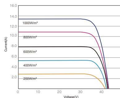
昊宇光伏I-V曲线图(555W)
