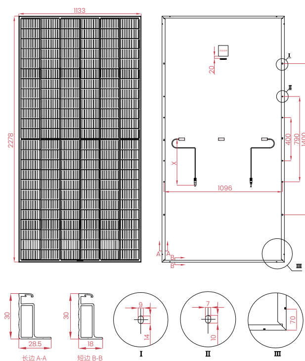
工程图纸
