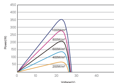
昊宇光伏 P-V 曲线图(350W)
