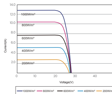
昊宇光伏 I-V 曲线图(350W)
