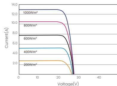
昊宇光伏I-V曲线图(365W)
