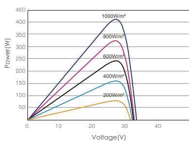
昊宇光伏P-V曲线图(410W)
