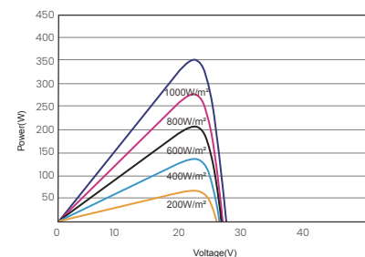
昊宇光伏 P-V 曲线图(350W)
