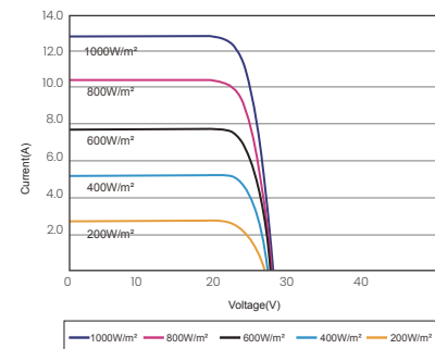
昊宇光伏 I-V 曲线图(350W)
