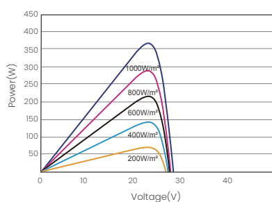
昊宇光伏P-V曲线图(360W)
