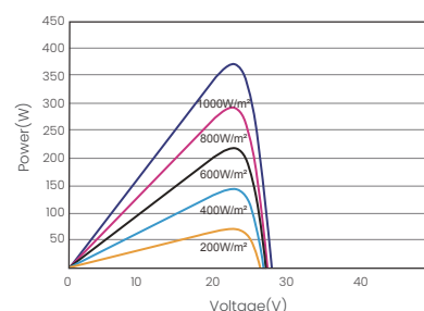
昊宇光伏P-V曲线图(365W)
