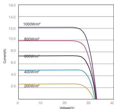
昊宇光伏电流-电压曲线图(510W)
