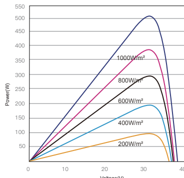
昊宇光伏功率-电压曲线图(510W)
