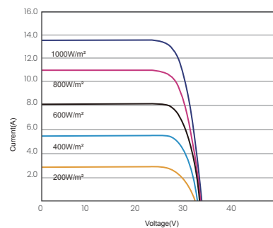
昊宇光伏I-V曲线图(430W)
