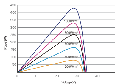
昊宇光伏P-V曲线图(430W)
