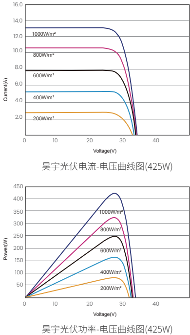
IV 曲线图
