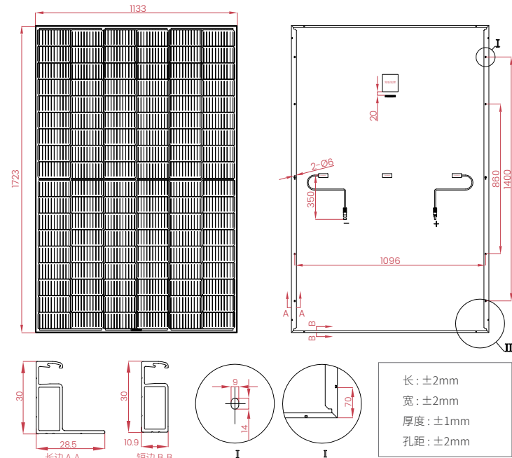
工程图纸
