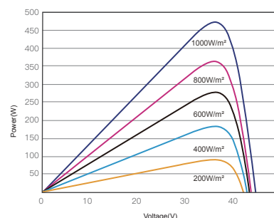
昊宇光伏P-V曲线图(475W)
