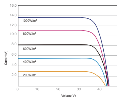
昊宇光伏I-V曲线图(475W)
