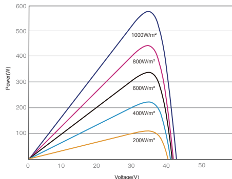
昊宇光伏P-V曲线图(580W)
