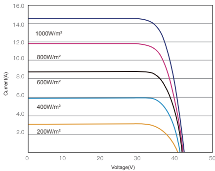
昊宇光伏I-V曲线图(595W)
