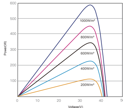
昊宇光伏P-V曲线图(595W)
