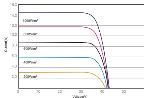
昊宇光伏I-V曲线图(585W)
