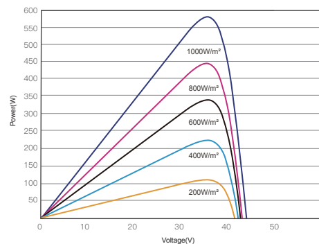
昊宇光伏P-V曲线图(585W)
