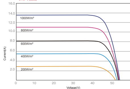
昊宇光伏 I-V 曲线图(575W)
