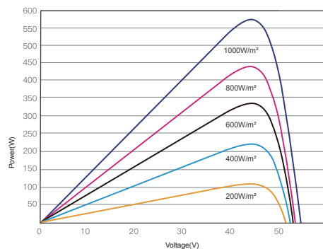
昊宇光伏 P-V 曲线图(575W)
