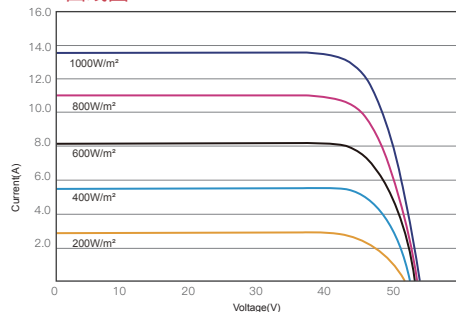
昊宇光伏 I-V 曲线图(575W)
