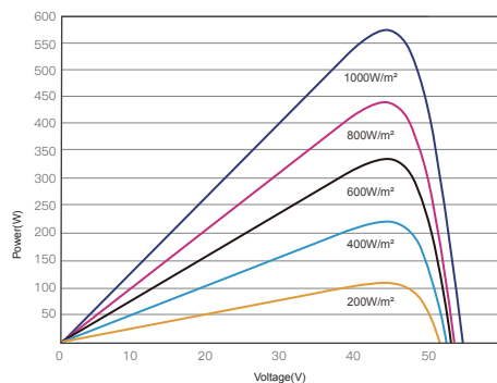
昊宇光伏 P-V 曲线图(575W)
