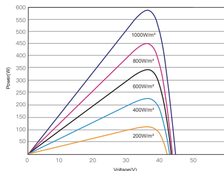
昊宇光伏 P-V 曲线图(590W)
