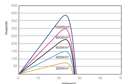
昊宇光伏P-V曲线图(385W)
