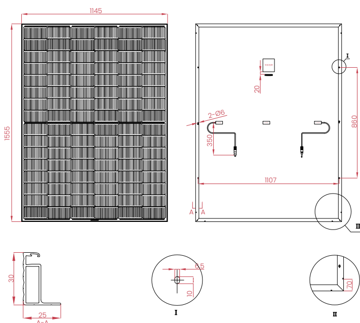
工程图纸
