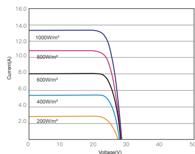
昊宇光伏I-V曲线图(385W)
