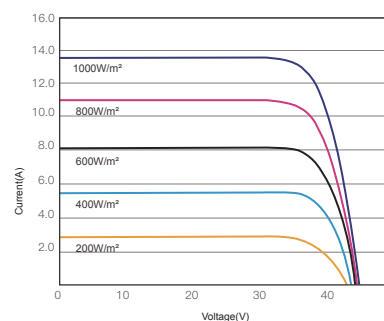
昊宇光伏I-V曲线图(475W)
