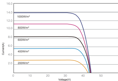
昊宇光伏I-V曲线图(570W)
