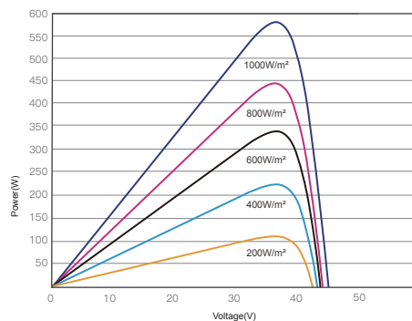
昊宇光伏P-V曲线图(570W)
