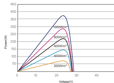
昊宇光伏P-V曲线图(370W)
