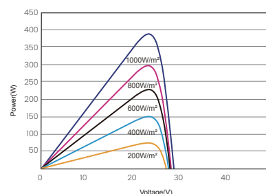
昊宇光伏P-V曲线图(380W)
