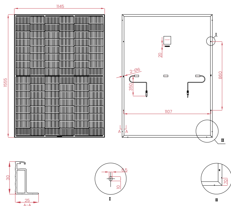
工程图纸
