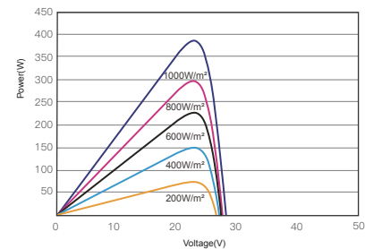
昊宇光伏P-V曲线图(385W)
