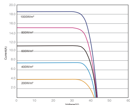
昊宇光伏I-V曲线图(595W)
