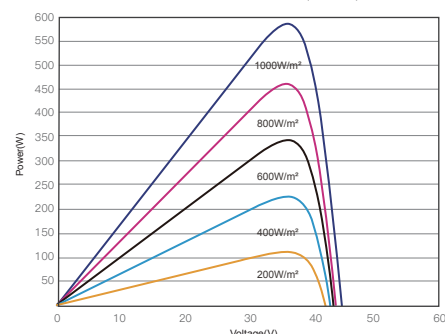
昊宇光伏P-V曲线图(595W)
