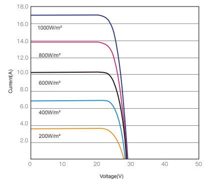
昊宇光伏I-V曲线图(395W)
