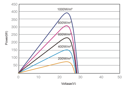
昊宇光伏P-V曲线图(395W)
