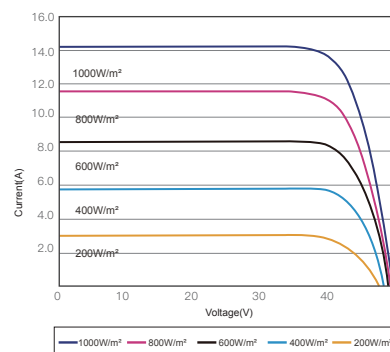
昊宇光伏I-V曲线图(550W)
