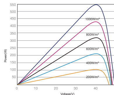
昊宇光伏P-V曲线图(550W)
