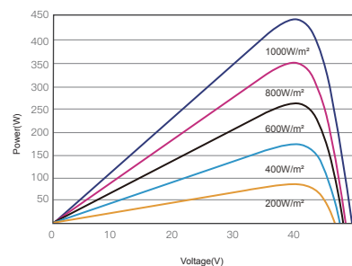
昊宇光伏P-V曲线图(445W)
