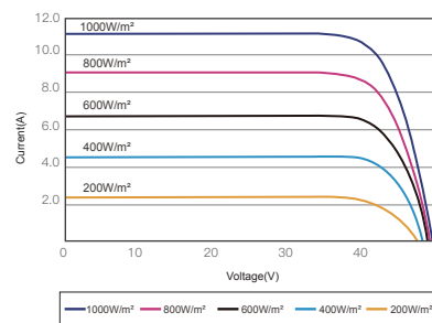
昊宇光伏I-V曲线图(445W)
